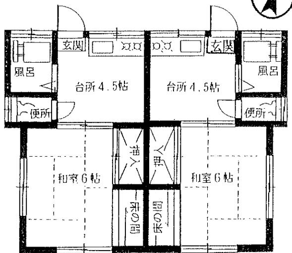
102 【1階平面図】
