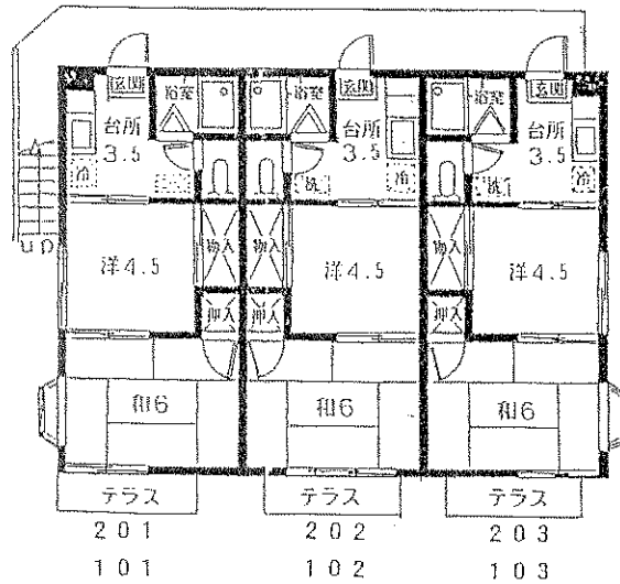
1階2階平面図
