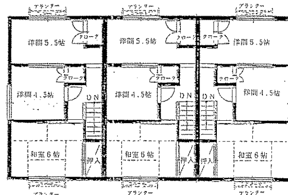
【2階平面図】
