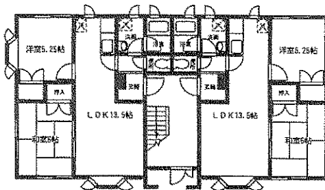
1 階平面図 101号
