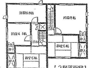
【2階平面図】
