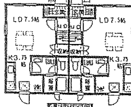
1階平面図
